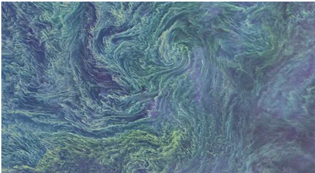
Detalj ur satellitfoto av cyanobakterieblomning i centrala Östersjön, 11 augusti 2015. Bildens längsida är cirka 100 kilometer. Det raka vita strecket upptill till vänster i bilden är kondensstrimma efter ett flygplan. Foto: © NASA Earth Observatory.
